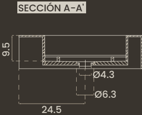
SENO DERECHA RECTO · STRAIGHT RIGHT SINK
