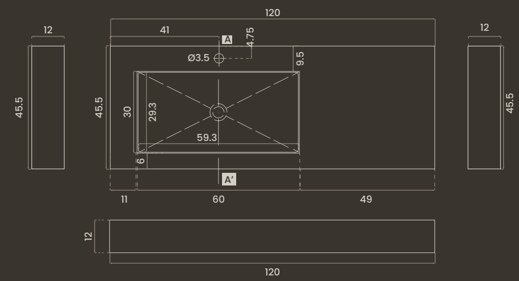
SENO IZQUIERDA RECTO · STRAIGHT LEFT SINK
