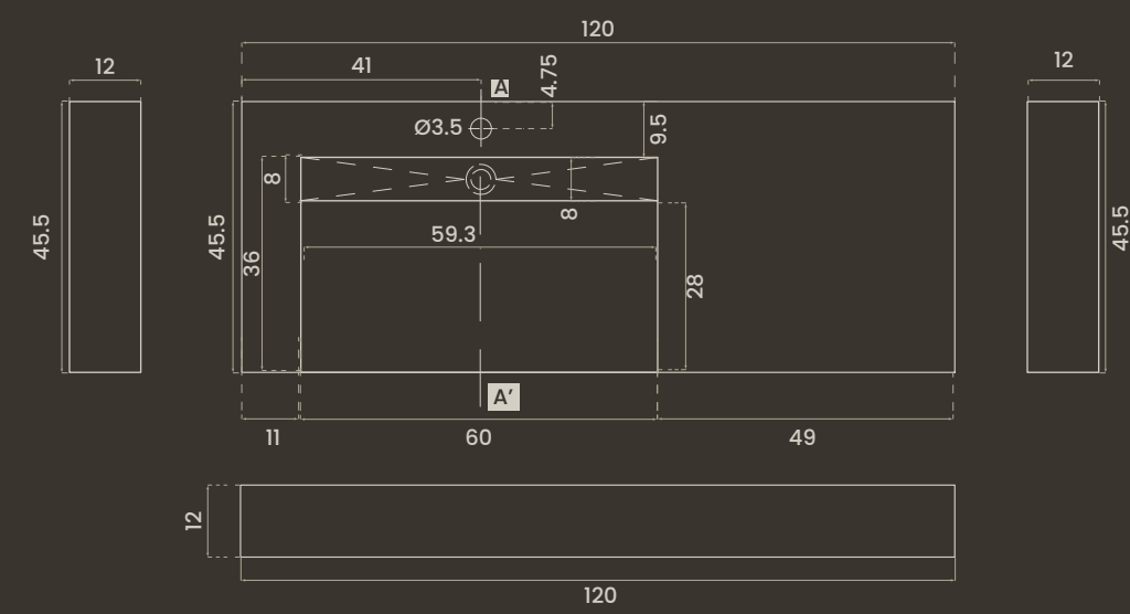
SENO IZQUIERDA RAMPA · INCLINED LEFT SINK
