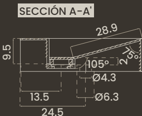
SENO DERECHA RAMPA · INCLINED RIGHT SINK
