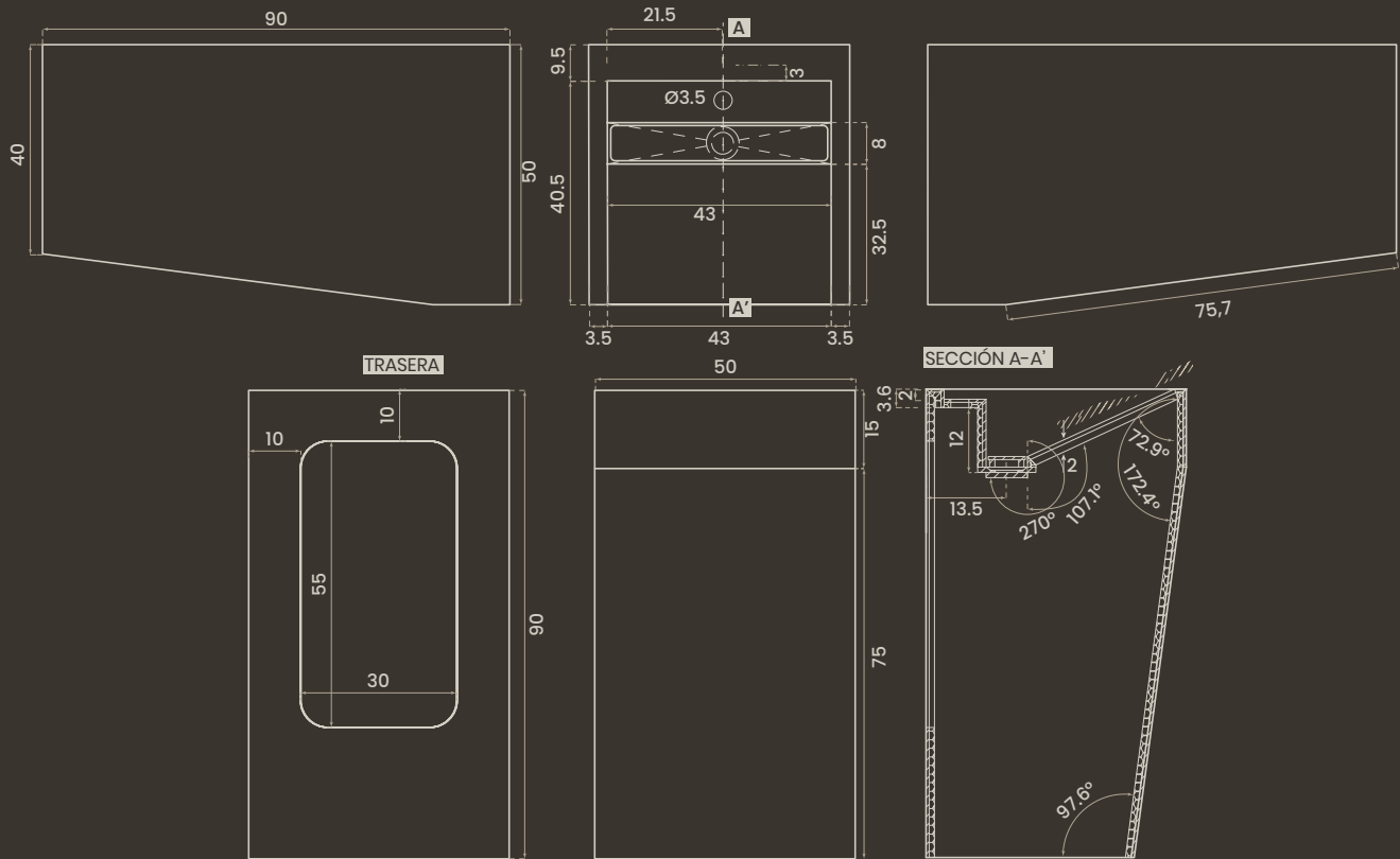
SENO RECTO · STRAIGHT SINK
