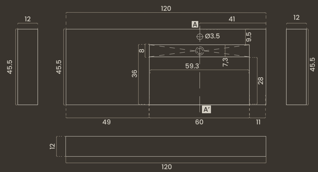
SENO DERECHA RAMPA · INCLINED RIGHT SINK
