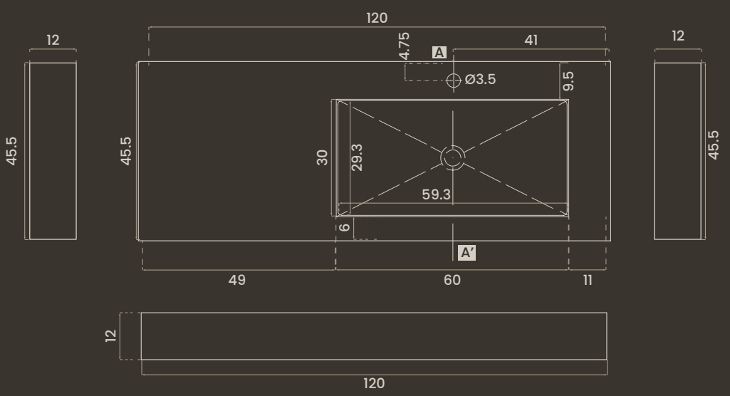
SENO DERECHA RECTO · STRAIGHT RIGHT SINK
