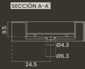
SENO RECTO · STRAIGHT SINK
