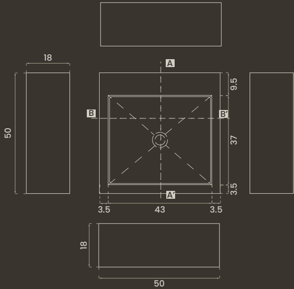
SENO RECTO · STRAIGHT SINK
